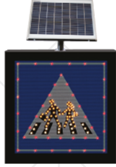
Güneş Enerjili Okul Geçidi Levhası AY-14b L-5077
